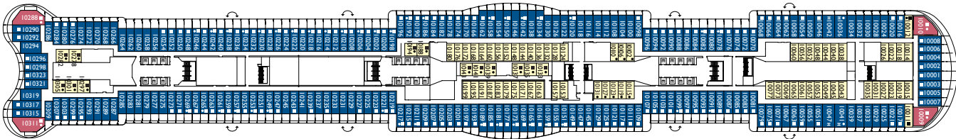
EXEMPLARISCHER DECKPLAN FÜR DIE DECKS 10 ROMA, DECK 11 FIRENZE, DECK 12 GENOVA, DECK 14 VENEZIA UND DECK 15 MILANO
